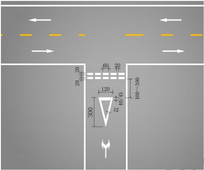
图 D.3 减速让标线（单位：cm）
