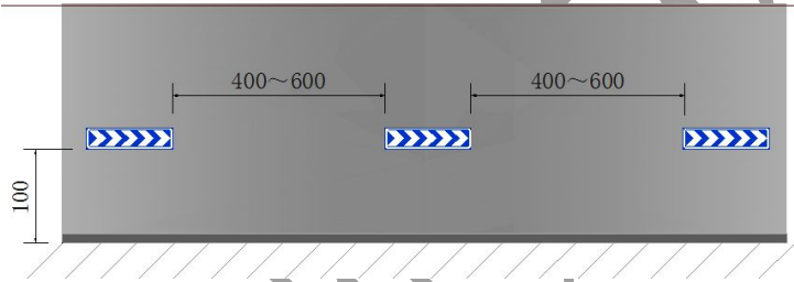
图B. 21 线形诱导标（单位：cm）
