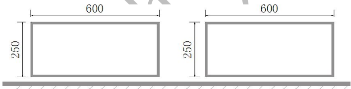
图 D.9 c) 平行式停车位车位线（单位：cm）
