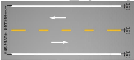
图 D. 6 a) 双向车行道黄色虚线分界线（单位：mm）
