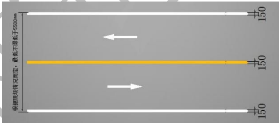
图 D. 6 b) 双向车行道黄色实线分界线（单位：mm）
