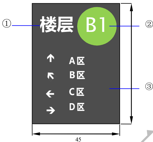
图B. 18 停车楼层及区域指向标志牌示意及推荐尺寸（单位：cm）
