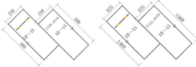
图 D.9 b) 倾斜式停车位车位线（单位：cm）
