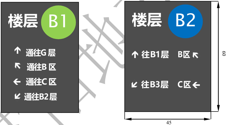
图B. 19 停车楼层及区域指向标志牌示意及推荐尺寸（单位：cm）
