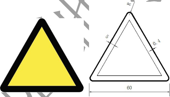
图B.1 警告标志底板及规格尺寸（单位：cm）
