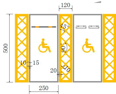
图 D. 12 无障碍机动车停车位（单位：cm）
