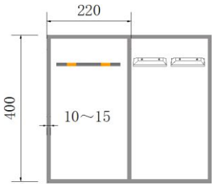
图 D.10 微型车位线（单位：cm）
