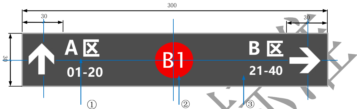
图B.11 停车区域引导标志牌示意及推荐尺寸（单位：cm）
