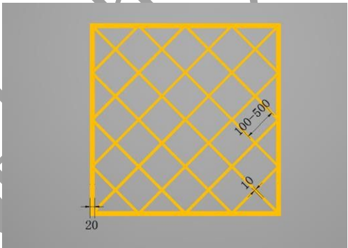
图 D.4 a) 网状线（单位：cm）
