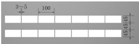
图 D.1 减速标线（单位：cm）
