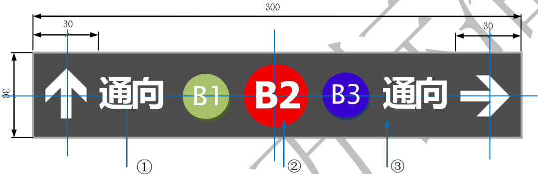
图B.15 停车楼层引导标志牌示意及推荐尺寸（单位：cm）
